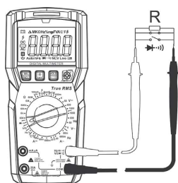
Рис. 7 Проверка целостности
