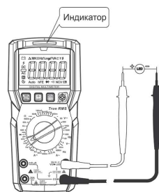
Рис. 14 Проверка светодиода
