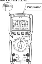
Рис. 13 Бесконтактное измерение напряжения
