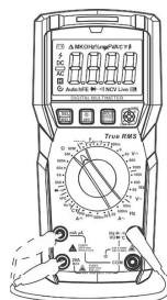
Рис. 6 Проверка предохранителей
