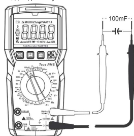
Рис. 9 Измерение ёмкости
