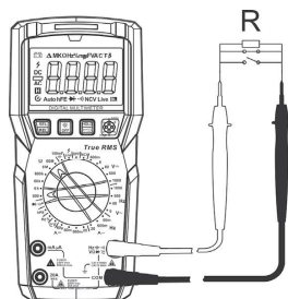
Рис. 5 Измерение сопротивления
