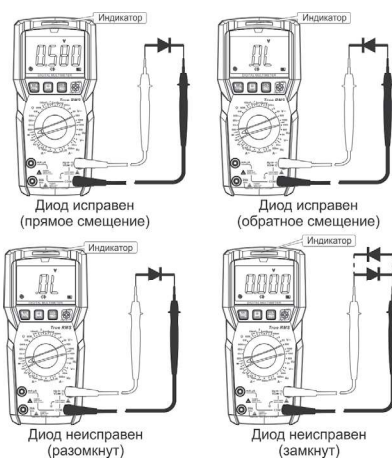
Рис. 8 Проверка диода
