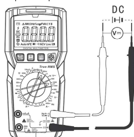
Рис. 3 Измерение напряжения постоянного тока
