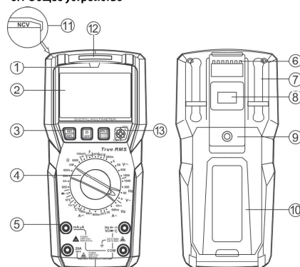
Рис. 1 Общее устройство
